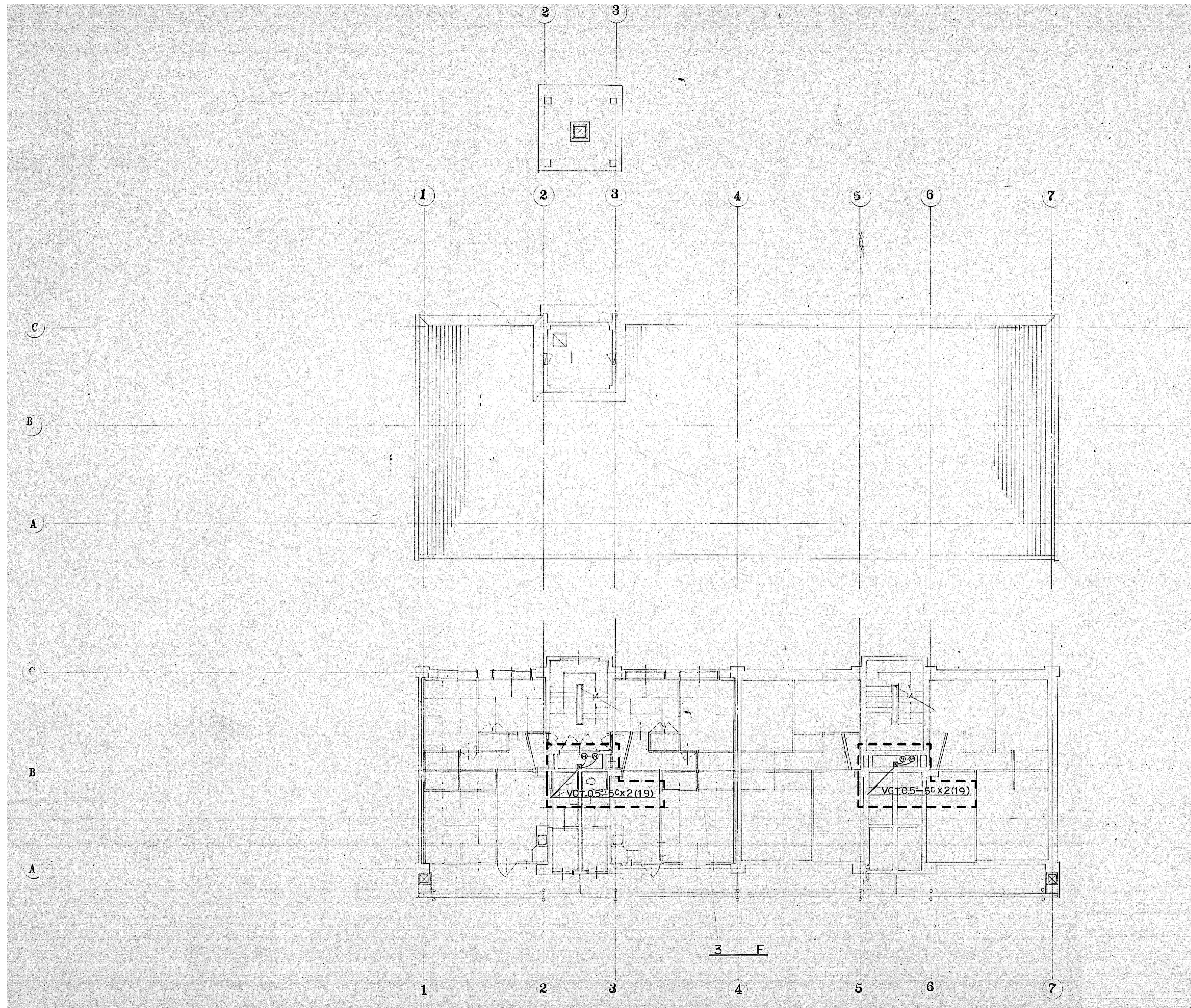
3 階 平面図 S=1/100
