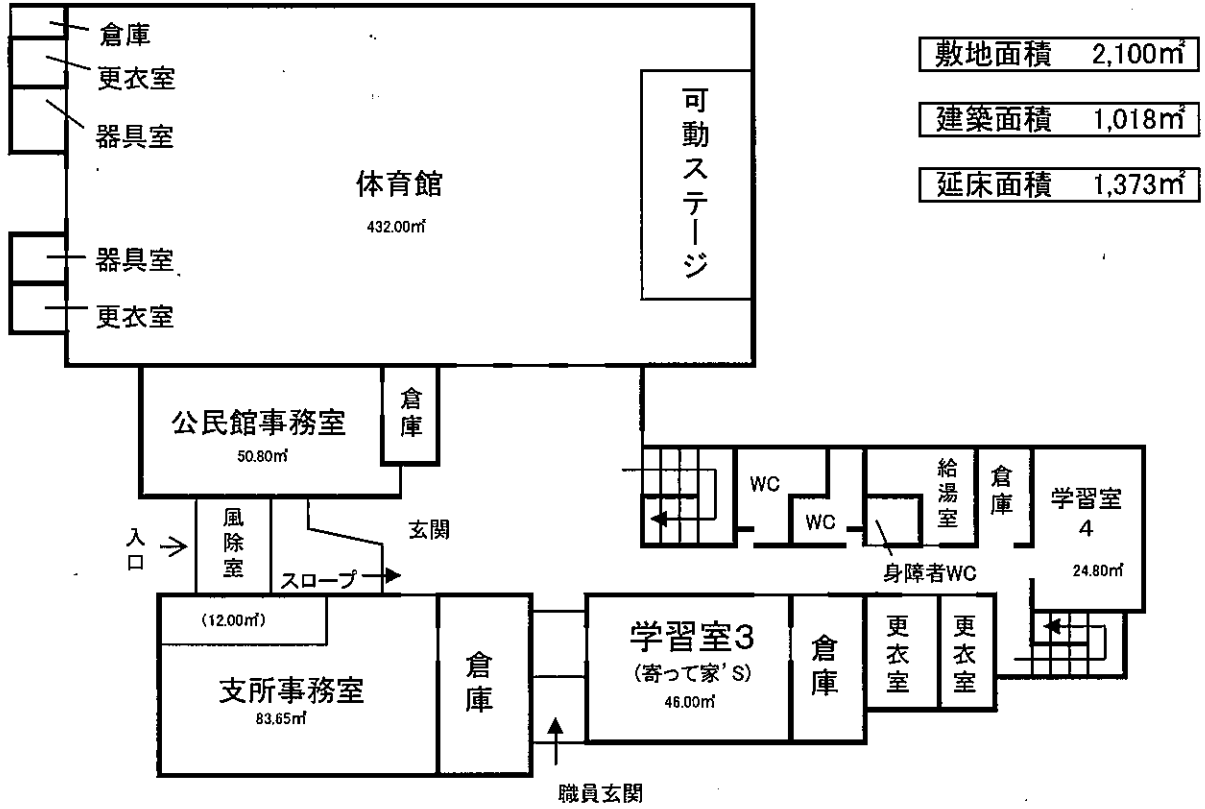
1階平面図
