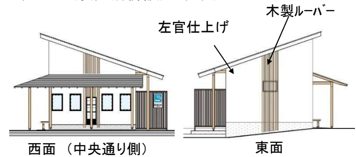
◇トイレ(喫煙所併設)立面図
