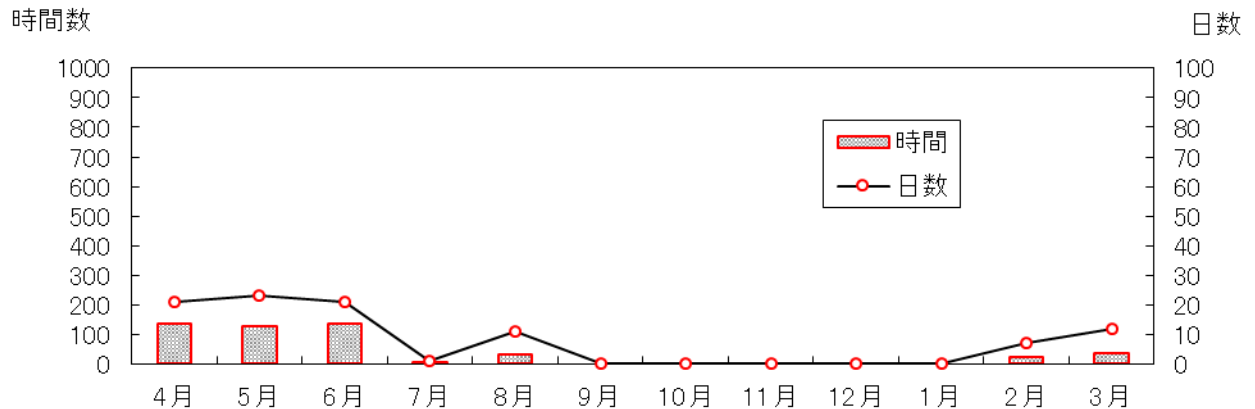
図2-11 月別光化学オキシダント*の環境基準*超過時間数と日数
