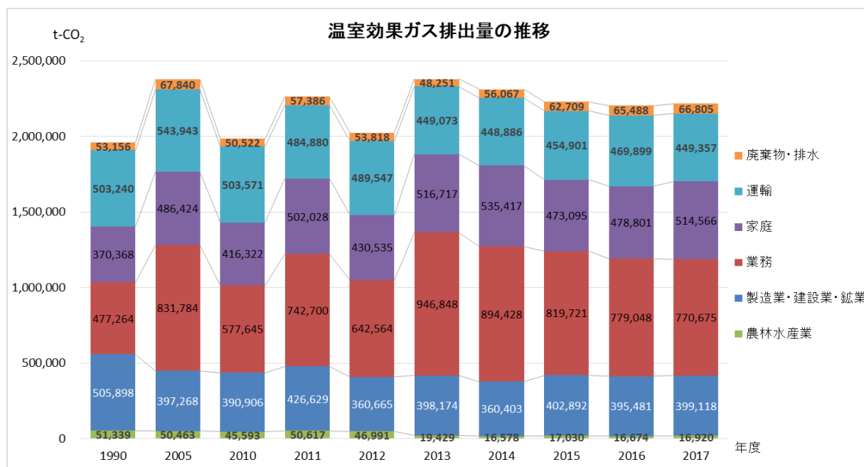
図 4-1 長野市域の温室効果ガス※排出量の推移
