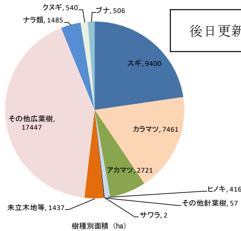
図2-14 長野市内の民有林の樹種構成
