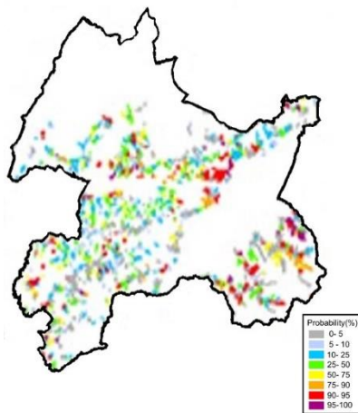
斜面崩壊発生確率 現在実績
