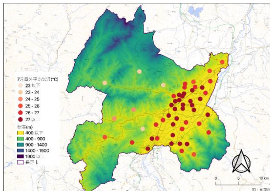
図 4-18 長野市内の小学校百葉箱内で測定された気温の分布図(2018年7月の月平均気温)
