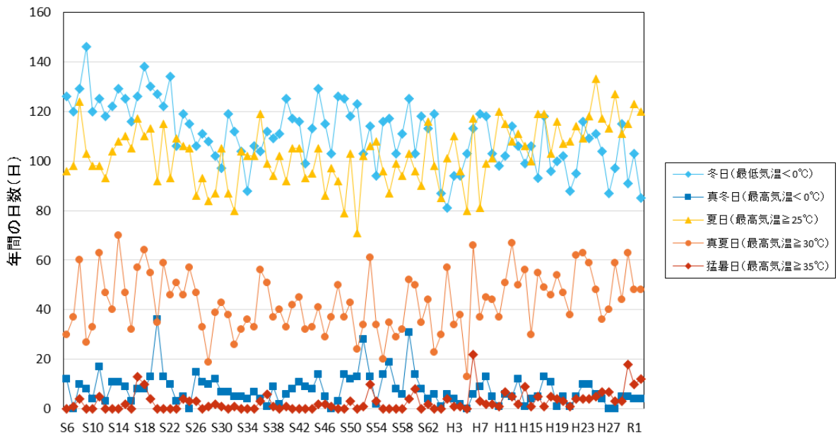
図 2-5 長野市内の冬日、夏日等の出現状況
