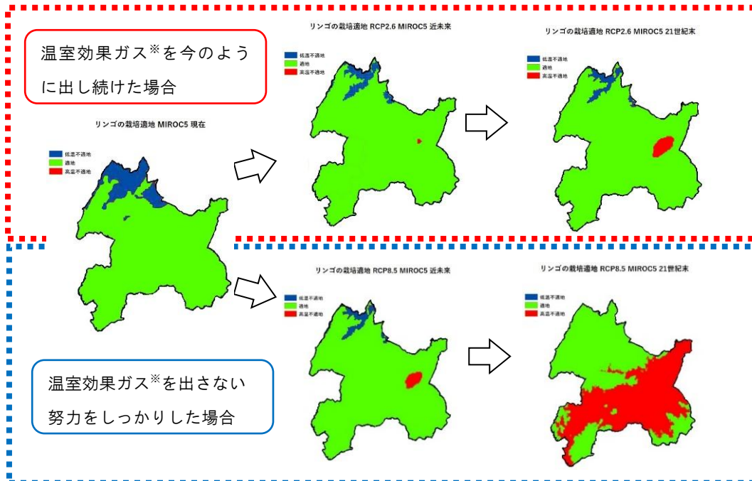
図 4-9 リンゴ栽培に適する年平均気温の予測シミュレーション
