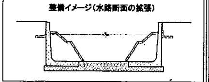
北八幡川改修後の河川断面イメージ(赤色部分)。傾斜護岸を直壁に改め、流量を確保(市森林農地整備課資料)
