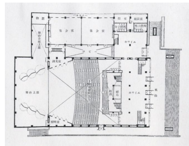
図1 長野市民会館2階平面図 「長野市民会館建設目論見書」より
