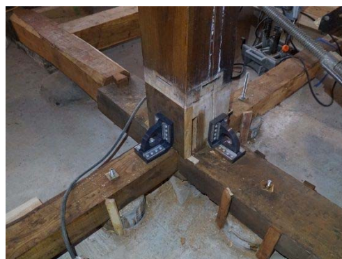
耐震補強工事(制震ダンパーの設置)
