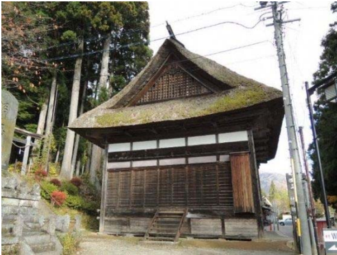
拝殿全景（修理前）
