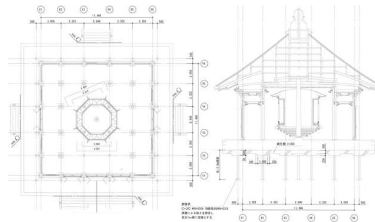
善光寺経蔵 平面図
