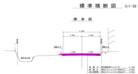
標準横断面図 (Standard Cross-section Diagram)
