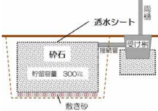
▼雨水浸透施設 設置例
