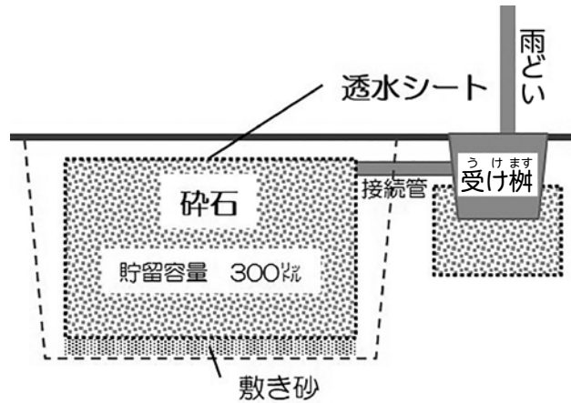
▲雨水浸透施設の設置例
